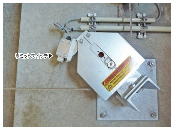
▲コーナーホイールユニット
