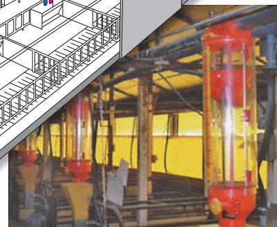
▲洗浄型ホッパーNK13B-04W
