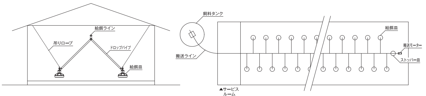
断面図
